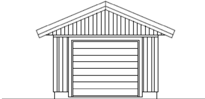
FASAD INFART
